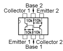
IMD3 (D3) (Q3020, 3021)
