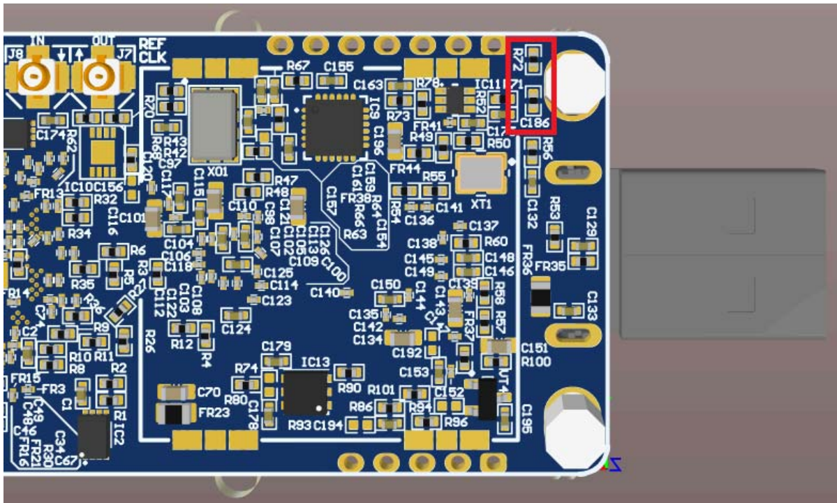
Figure 14: LimeSDR Mini v2.2 mounting hole clearence
