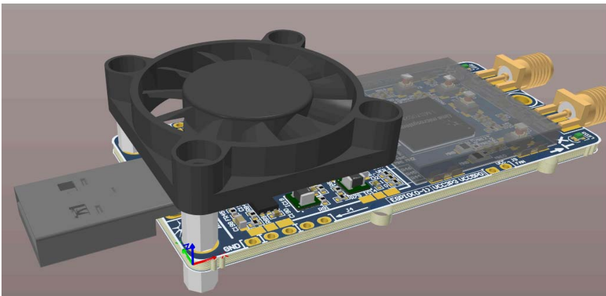
Figure 13: LimeSDR Mini v2.2 fan mounting
