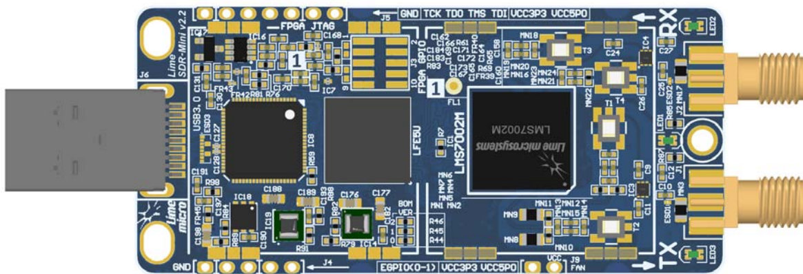
Figure 1: LimeSDR Mini v2.2 board top view
