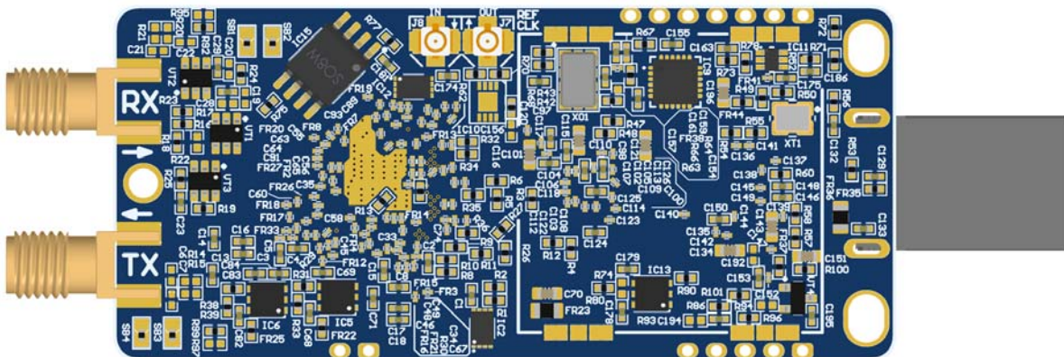
Figure 2: LimeSDR Mini v2.2 board bottom view
