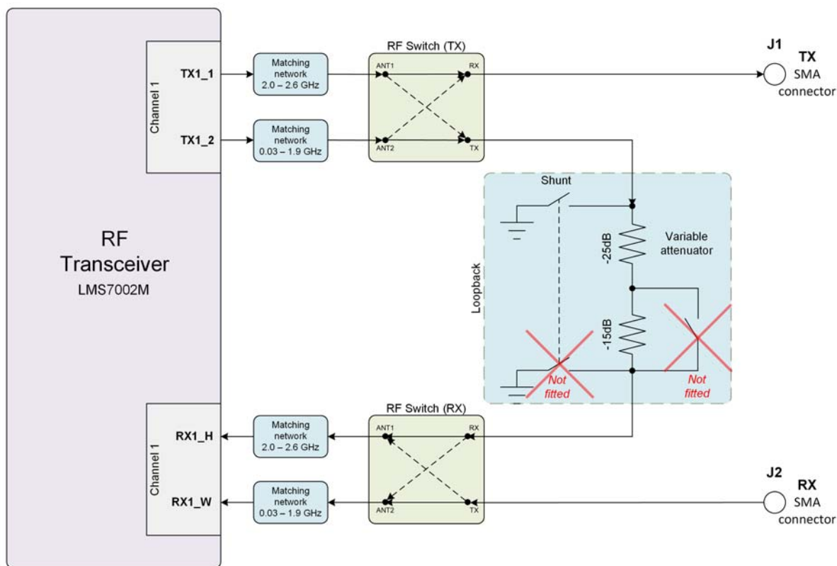
Figure 6: LimeSDR Mini v2.2 RF diagram
