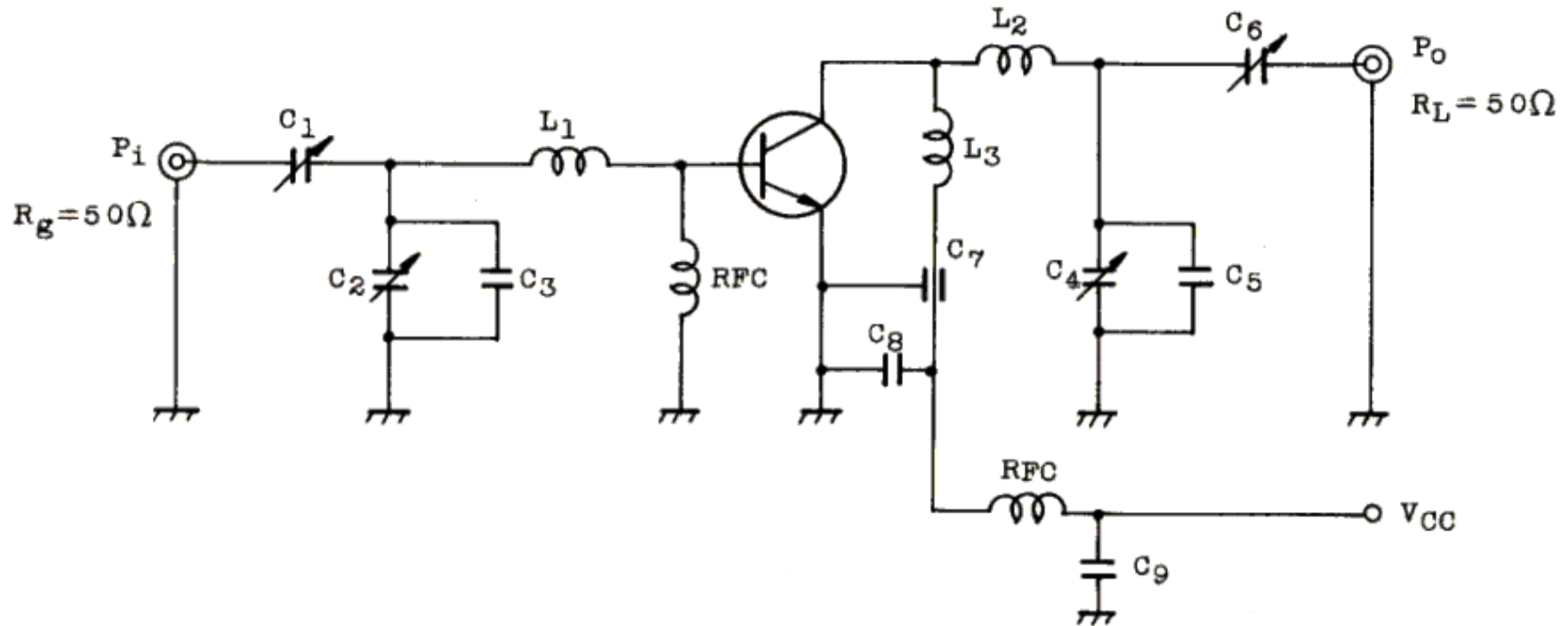
Fig. P_o TEST CIRCUIT
