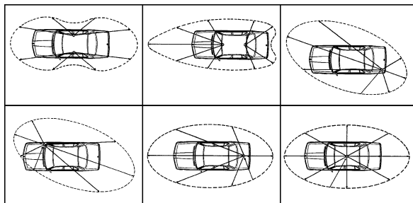
ANTENNEN-DIAGRAMM
