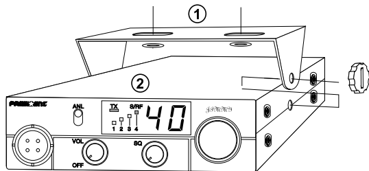
BEFESTIGUNG DES MONTAGEBÜGELS
