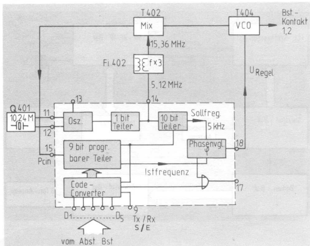
Bild 4 Blockschaltung der PLL-Einheit
