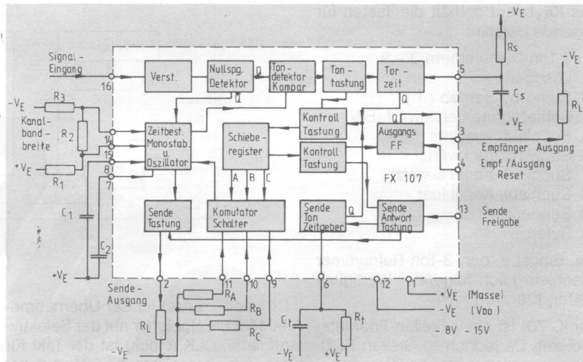
Bild 11 Blockschaltung des IC 620
