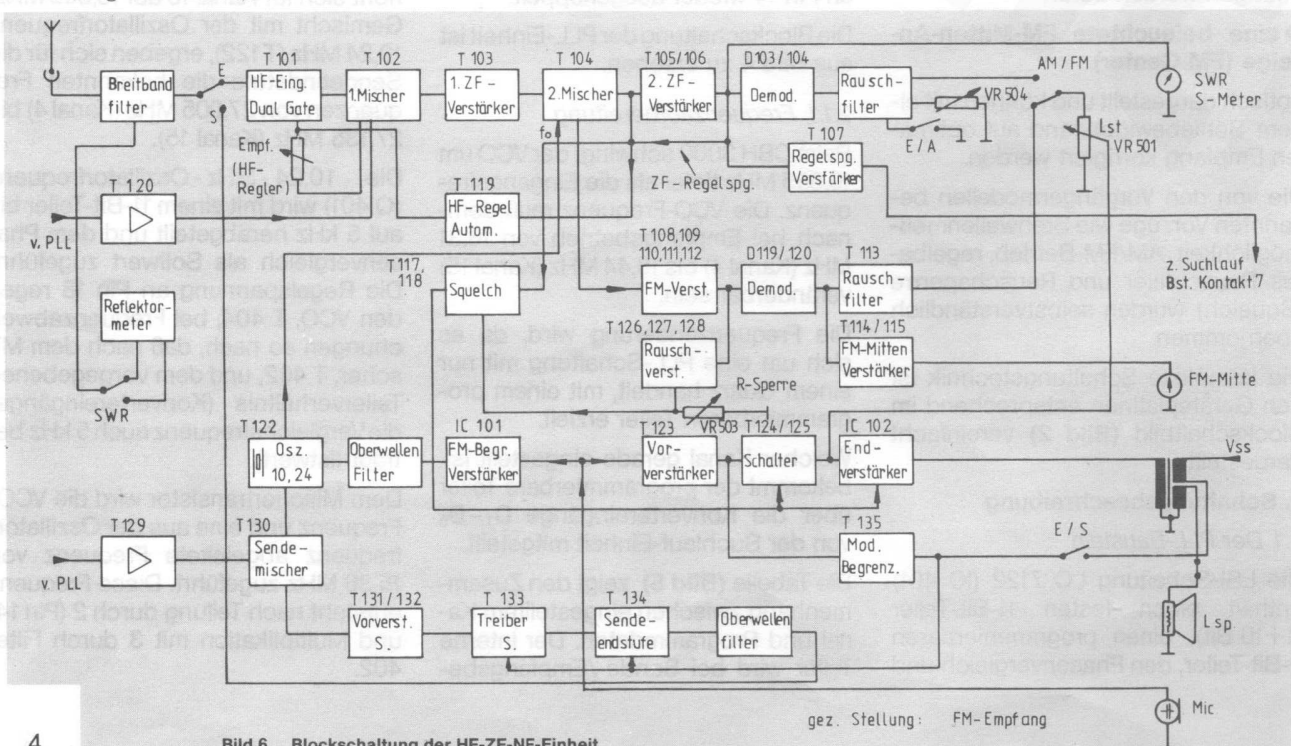
Bild 6 Blockschaltung der HF-ZF-NF-Einheit
