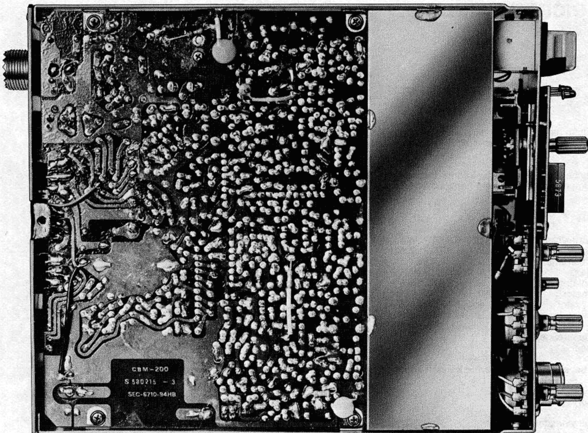
Lötansicht CBM 200
