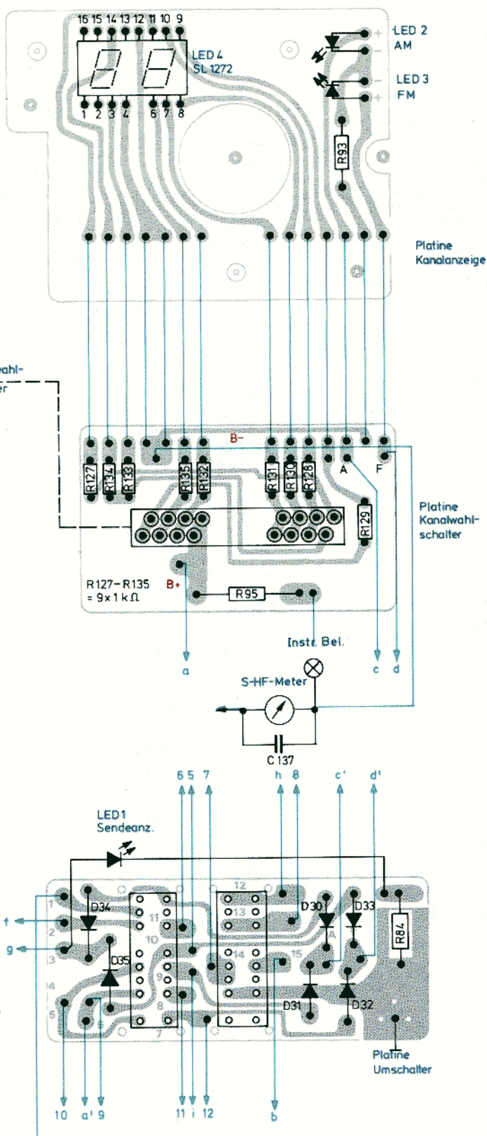
Druckschaltung mit Verdrahtung (Ansicht - Lötseite)
