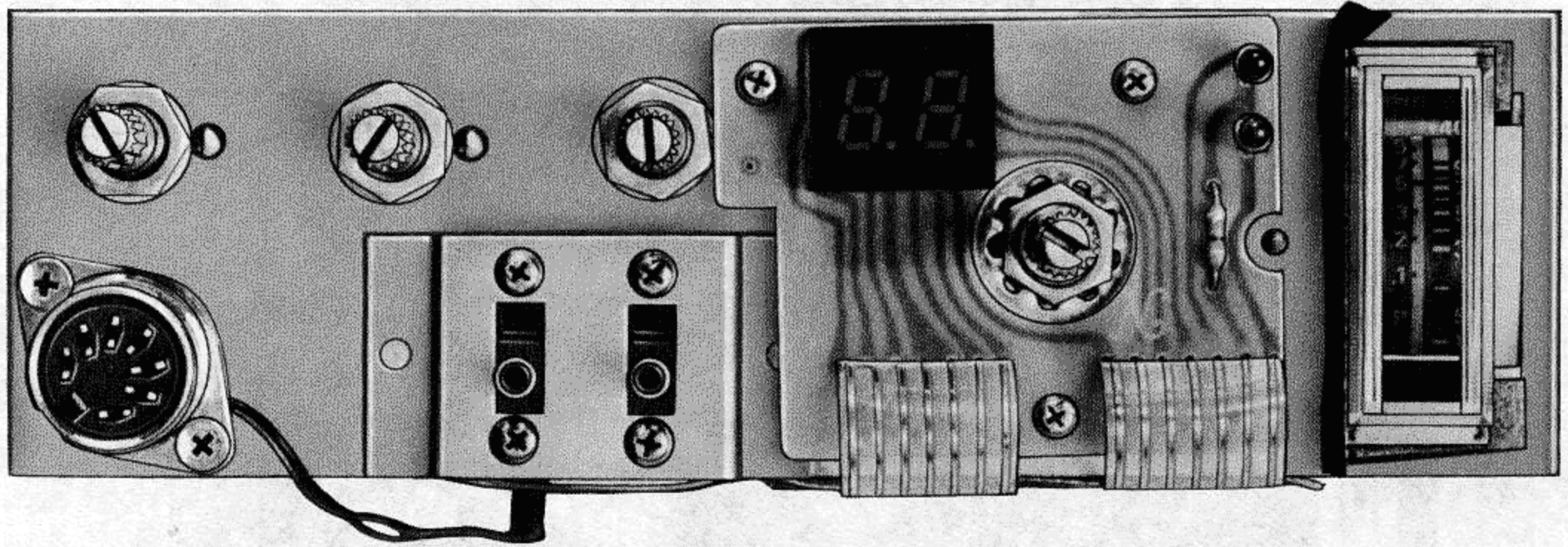
Frontansicht (Blende entfernt) CBM 200
