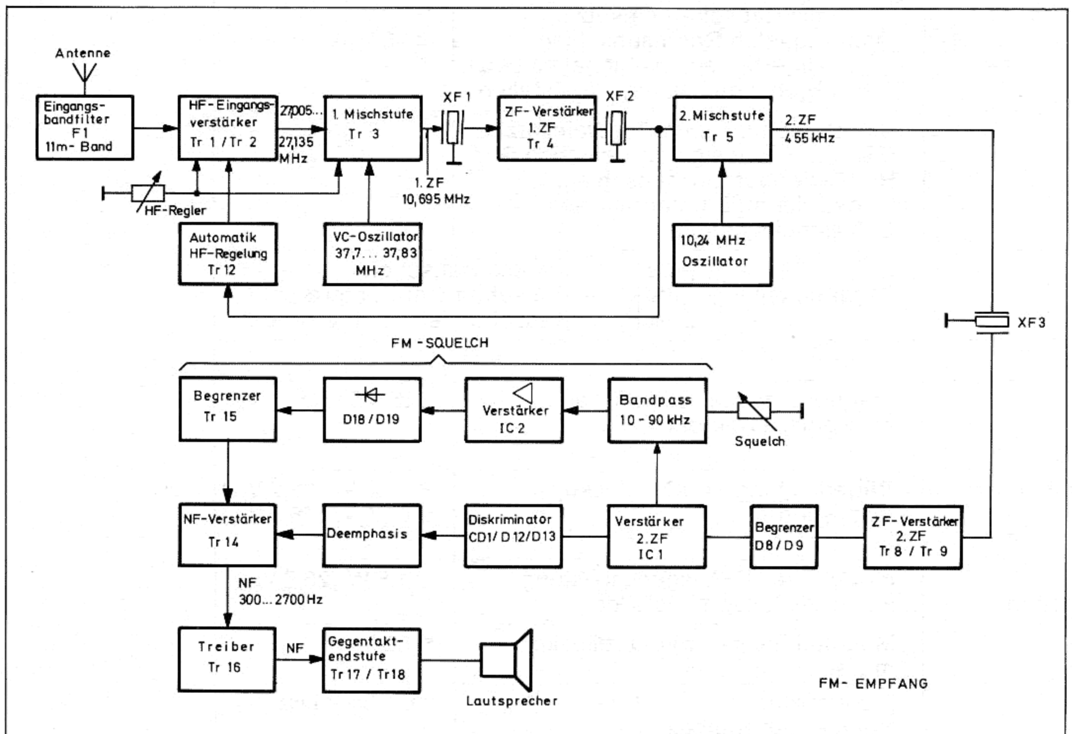
Blockschaltbild FM Empfang/Senden
