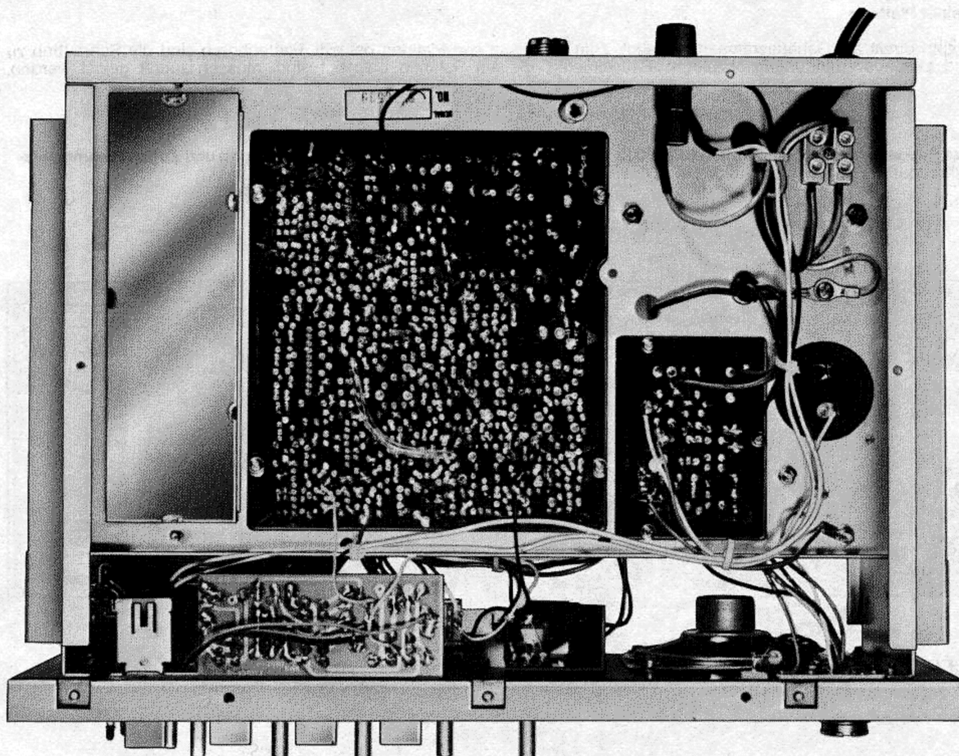
Lötansicht CBH 2000
