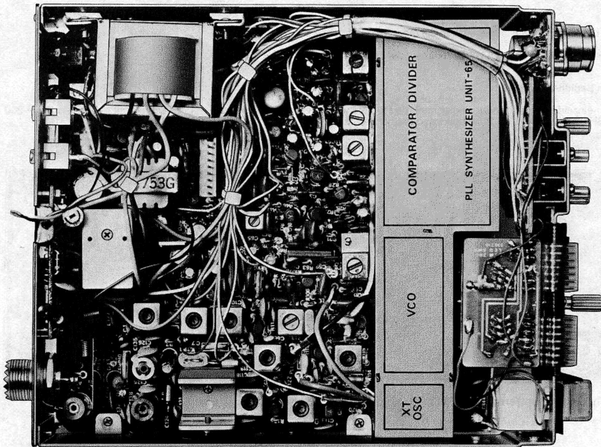
Gerätedraufsicht CBM 200
