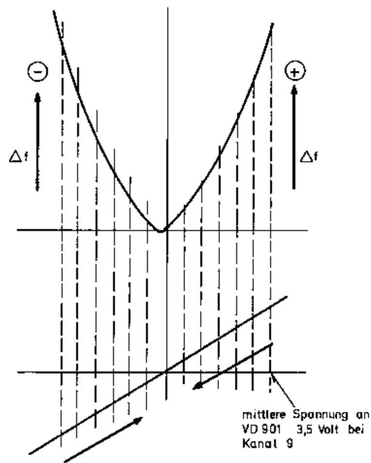
Spannung an VD 901
